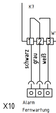
Abb. 8: Potentialfreier_Fernwarnkontakt_Schaltplan_PRO-ACTIVE
