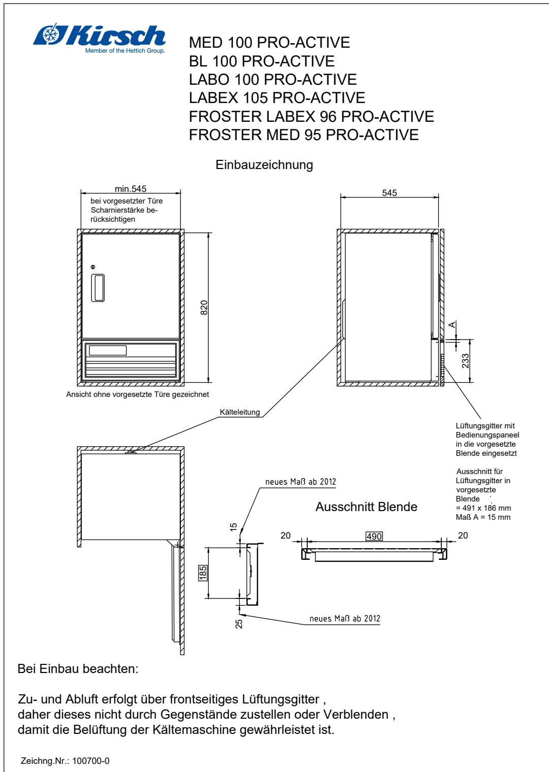
Abb. 9: Einbauzeichnung LABEX® 105 PRO-ACTIVE
