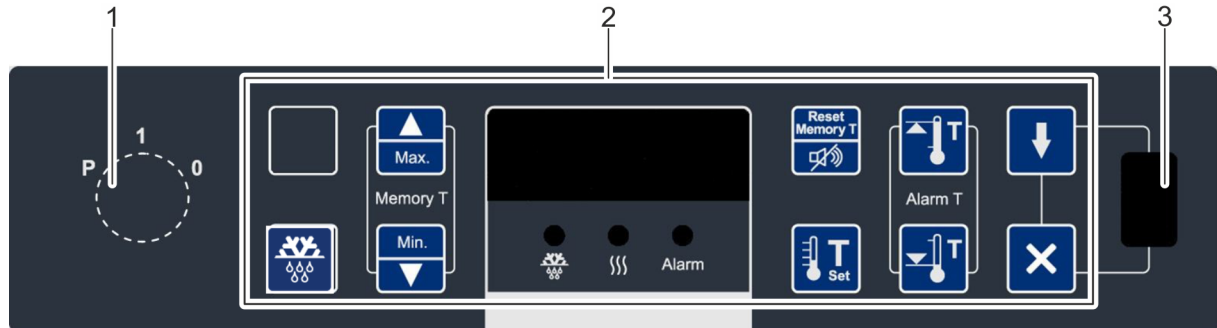
Abb. 2: Anzeige- und Bedieneinheit
