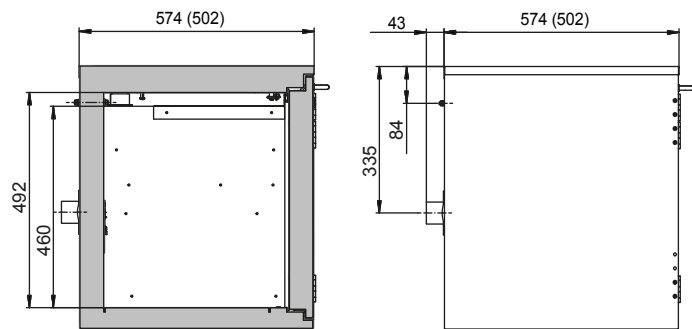
Draufsicht
