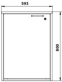
Frontalansicht
