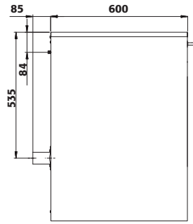
Seitenansicht
