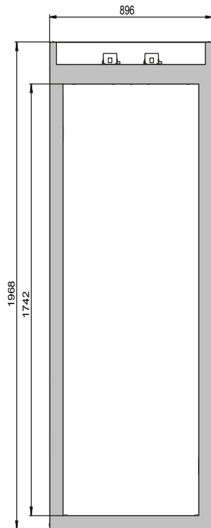
Frontalansicht
