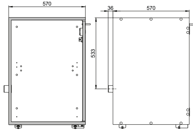
Seitenansicht
