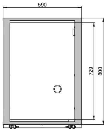
Frontalansicht
