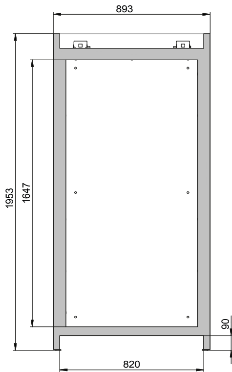
Frontalansicht
