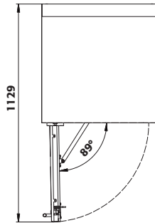
Draufsicht
