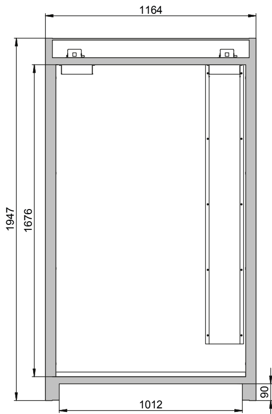
Frontalansicht
