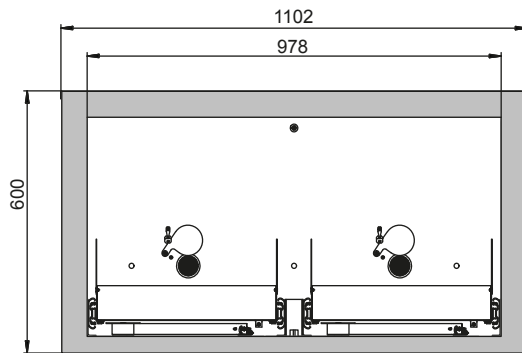
Frontalansicht
