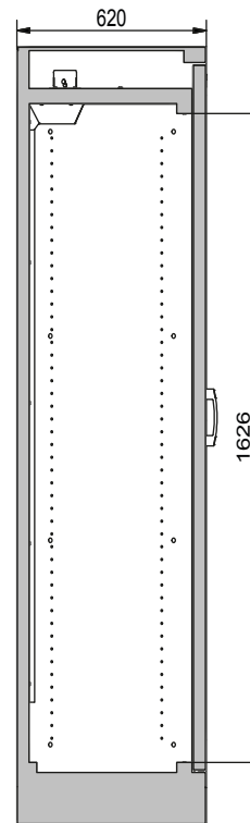
Seitenansicht
