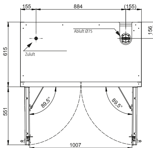
Draufsicht
