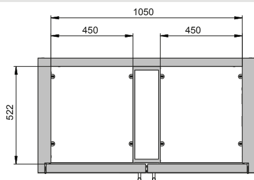
Draufsicht
