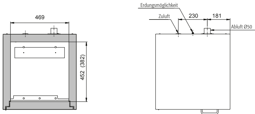
Draufsicht
