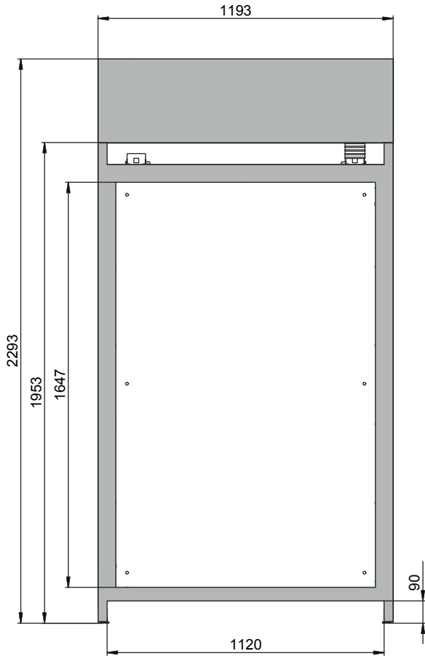
Frontalansicht
