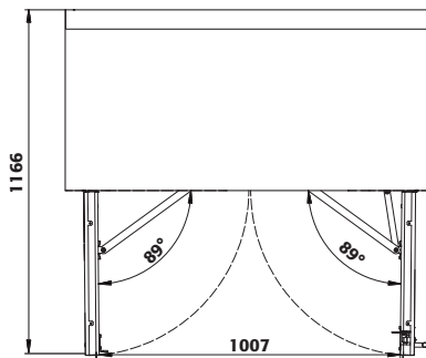
Draufsicht
