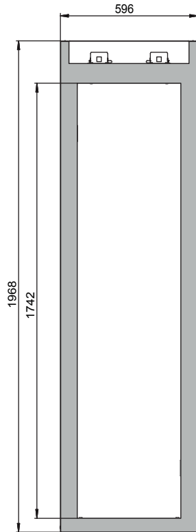
Frontalansicht
