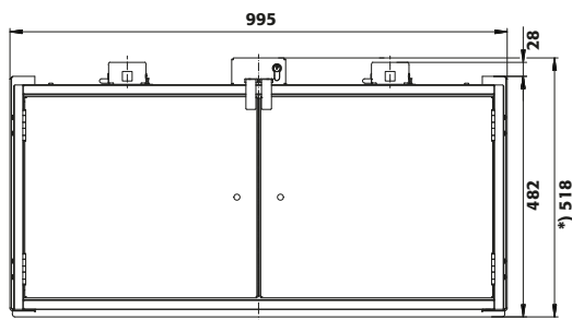
Frontalansicht
