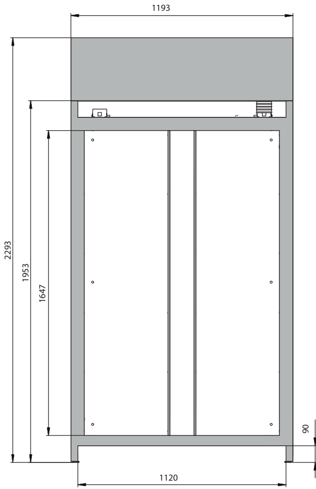
Frontalansicht
