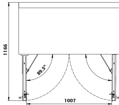
Draufsicht
