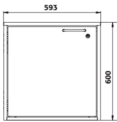
Frontalansicht
