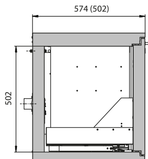
Draufsicht
