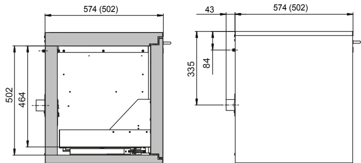
Draufsicht
